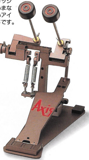
ツインペダル AX-TW ¥98,000 ツインペダルの弱点である左右のレスポンスの違いを見事に解消したツインペダルです。シングル同様ボールベアリングを多用し、スピード感あるプレイに差がでます。
